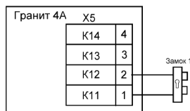
Рис. 2 Подключение электромагнитного замка
