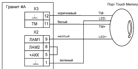
Рис. 1 Подключение порта Touch Memory
