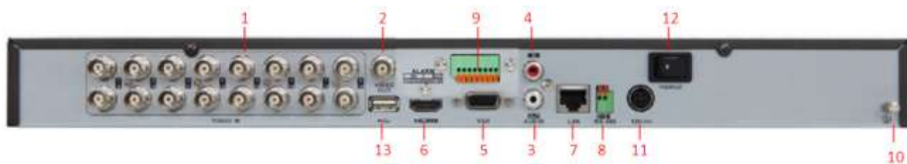
Рис.1.7.5. Задняя панель регистратора LTV-DVR-0861-HV и LTV-DVR-1662-HV
