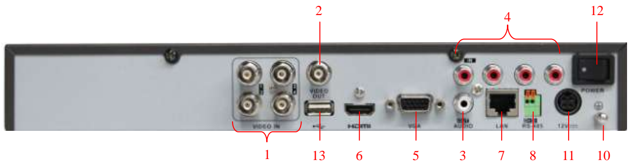
Рис.1.7.1. Задняя панель регистратора LTV-DVR-0432-HV
