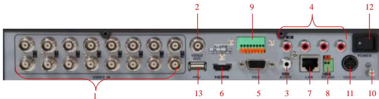
Рис.1.7.3. Задняя панель регистратора LTV-DVR-0831-HV
