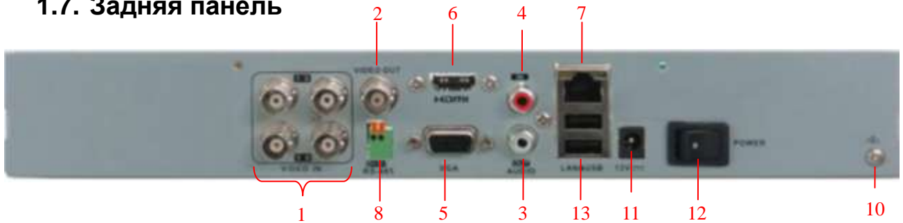
Рис.1.7.1. Задняя панель регистратора LTV-DVR-0432-HV
